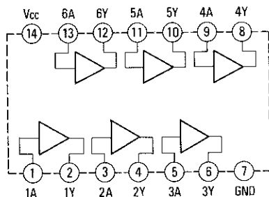
IC402 (SVIM53217P)
