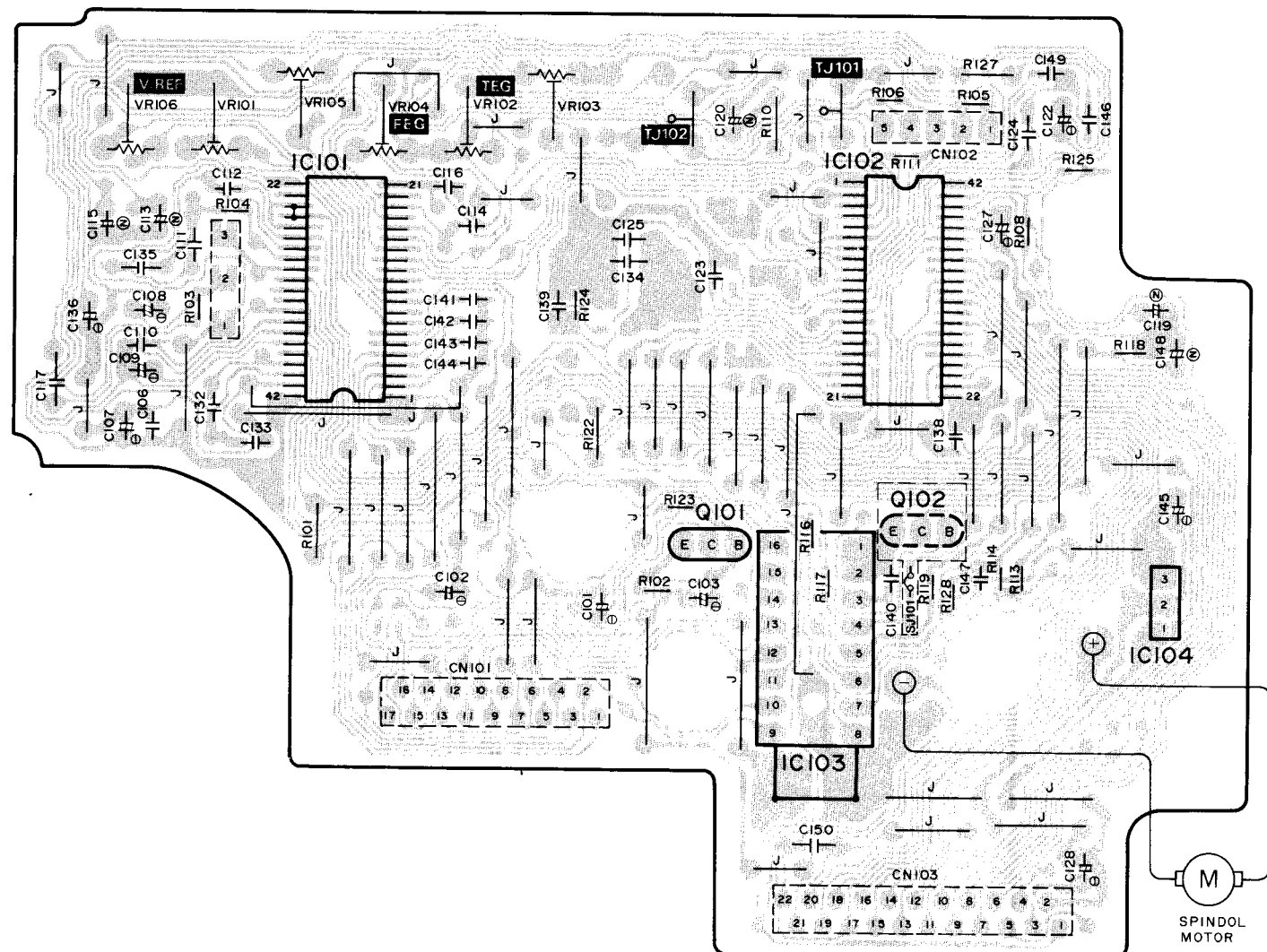
D SERVO P.C.B.
