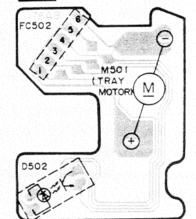
B TRAY MOTOR P.C.B. (REPI725A-N)
