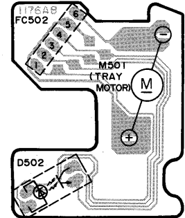
B TRAY MOTOR P.C.B. (REP I725A-N)
