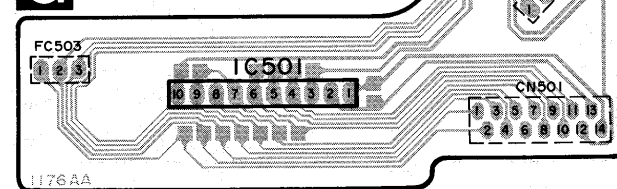
G SENSOR P.C.B.(REP I725A-N)
