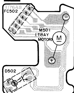
B TRAY MOTOR P.C.B. (REPI725A-N)
