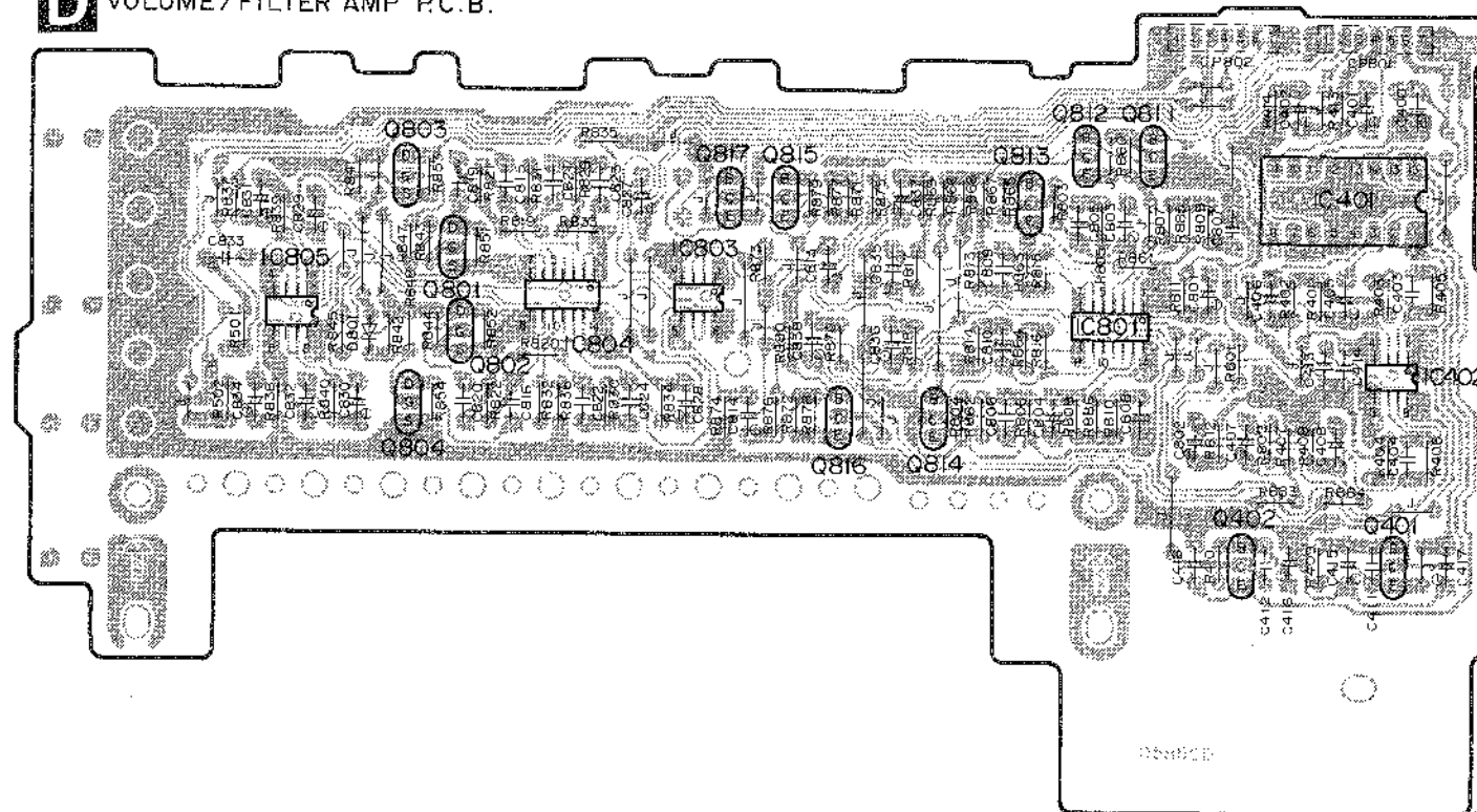
D VOLUME/FILTER AMP P.C.B.
