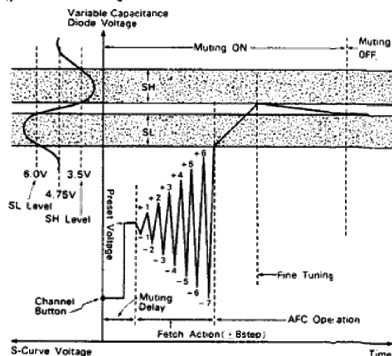
Fig.2-2 Preset Tuning
