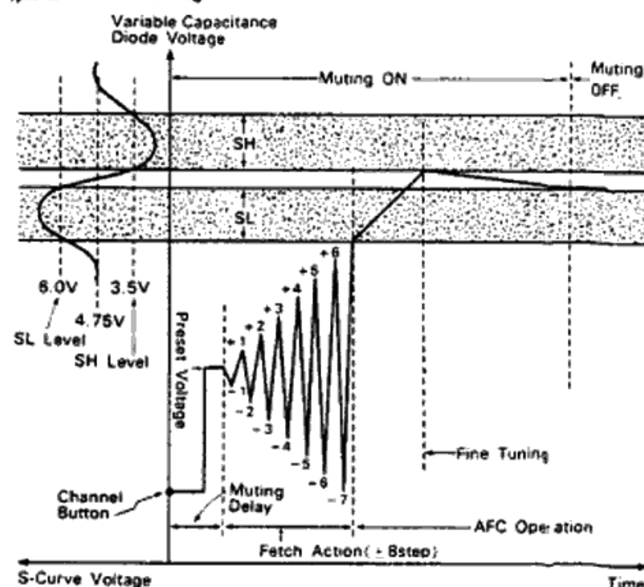
Fig.2-2 Preset Tuning
