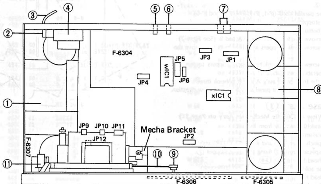
Parts List &lt;Front View&gt;
