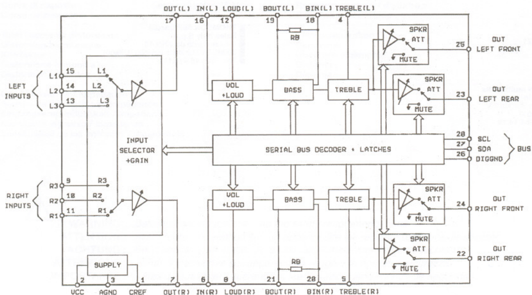
IC 401 TDA 7313
