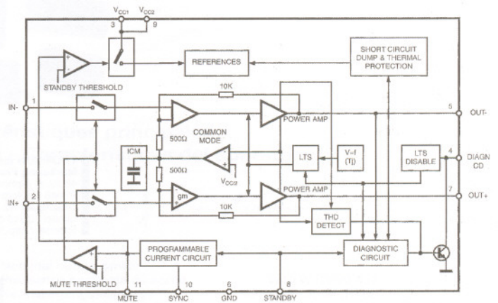
IC 802 TDA 7396
