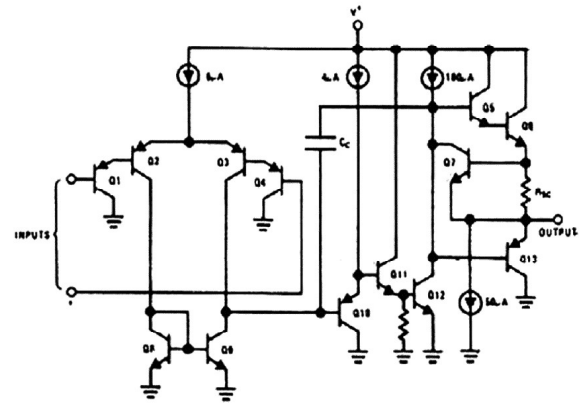
LM324
