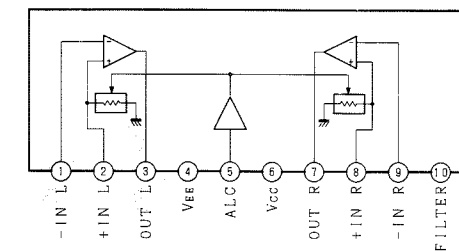
IC472 : HA12155 Dolby & Rec EQ Amp
