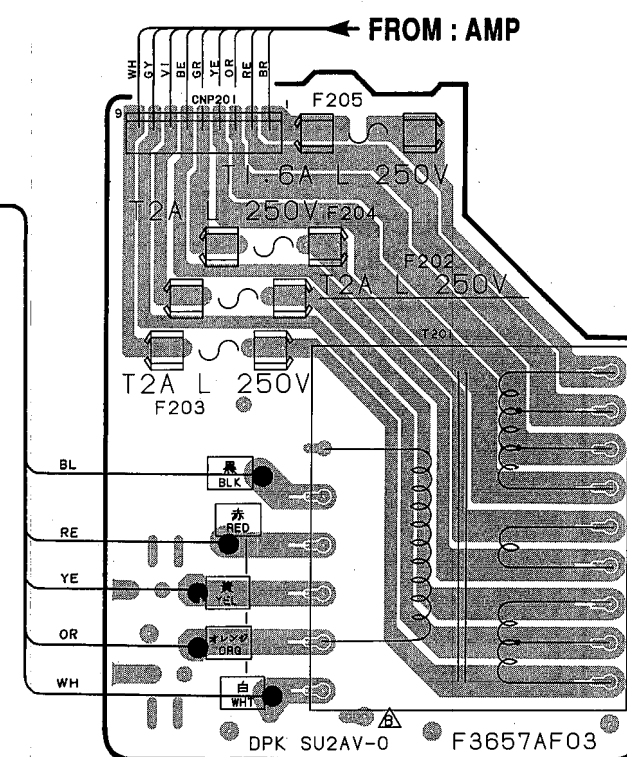
TRANS PWB ( PWB 201-3 )
