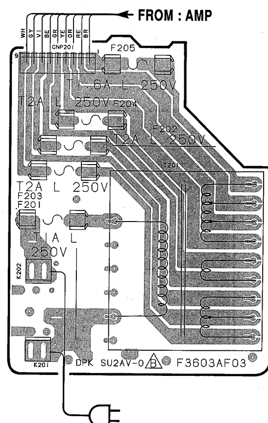
TRANS PWB ( PWB 201-3 )
