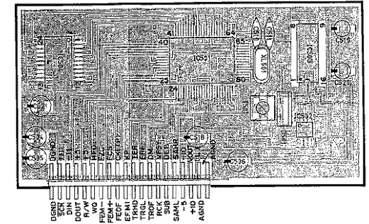
(Parts side)
