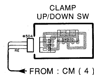
P.C.B. CM ( 2 )
