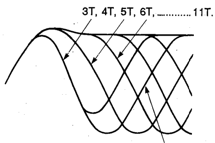
Waveforms 3T—11T.
