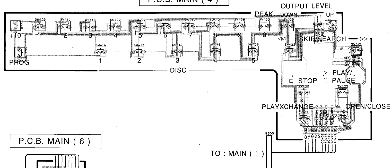
P.C.B. MAIN ( 4 )
