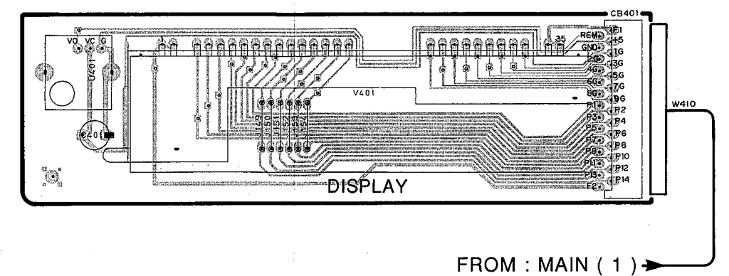
P.C.B. MAIN ( 5 )
