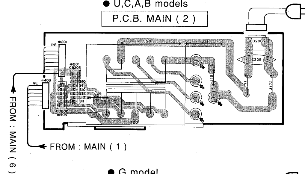
P.C.B. MAIN (2)
