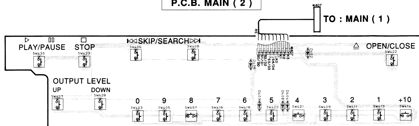
P.C.B. MAIN ( 2 )
