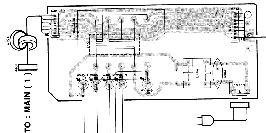
P.C.B. MAIN ( 4 )
