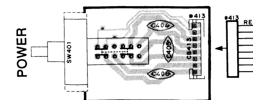
P.C.B. MAIN ( 5 )
