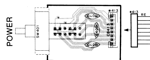
P.C.B. MAIN ( 5 )
