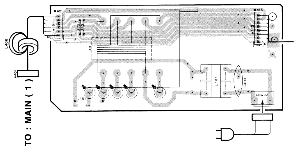
P.C.B. MAIN ( 4 )
