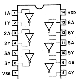
IC16 : PC74HCU04
