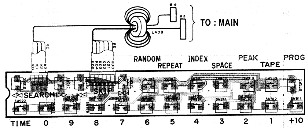
CDX-870 ROLLING SW P. C. B.
