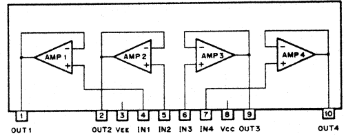
IC2, 15 : LB1641
