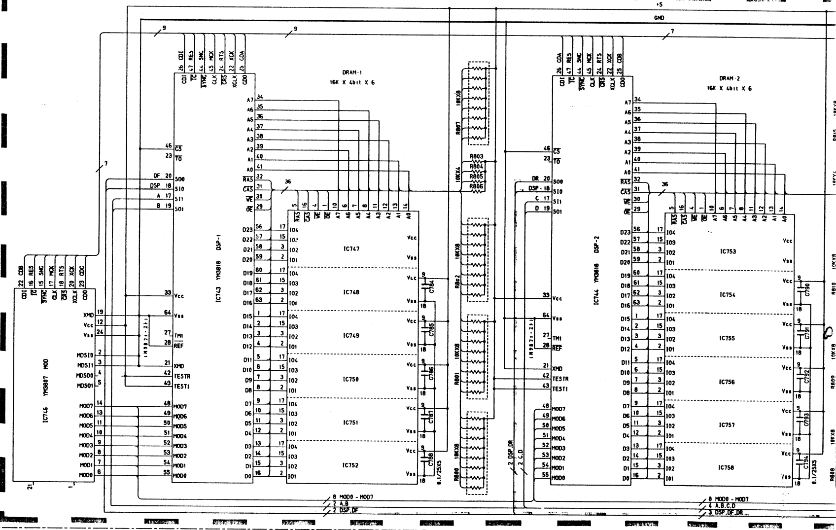
DSP UNIT
