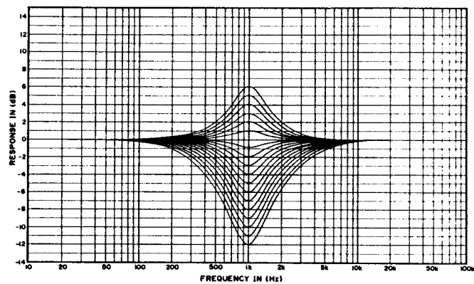
DEQ
