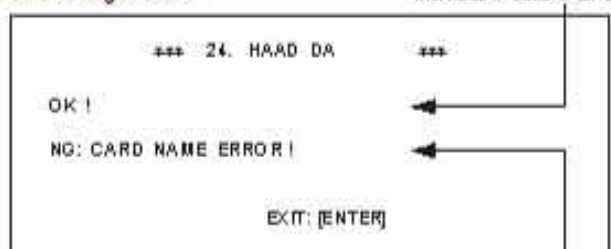
Fig. 46. HAAD DA REG Test Screen (2)
