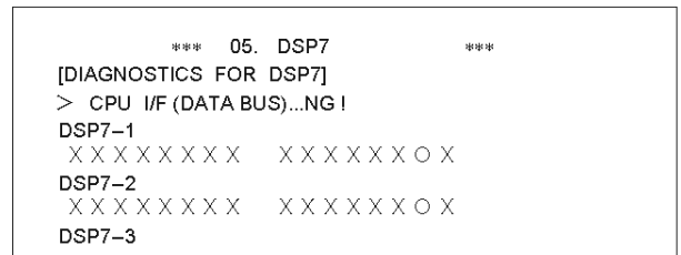
Fig. 17. DM DSP7 Test Screen (2)
