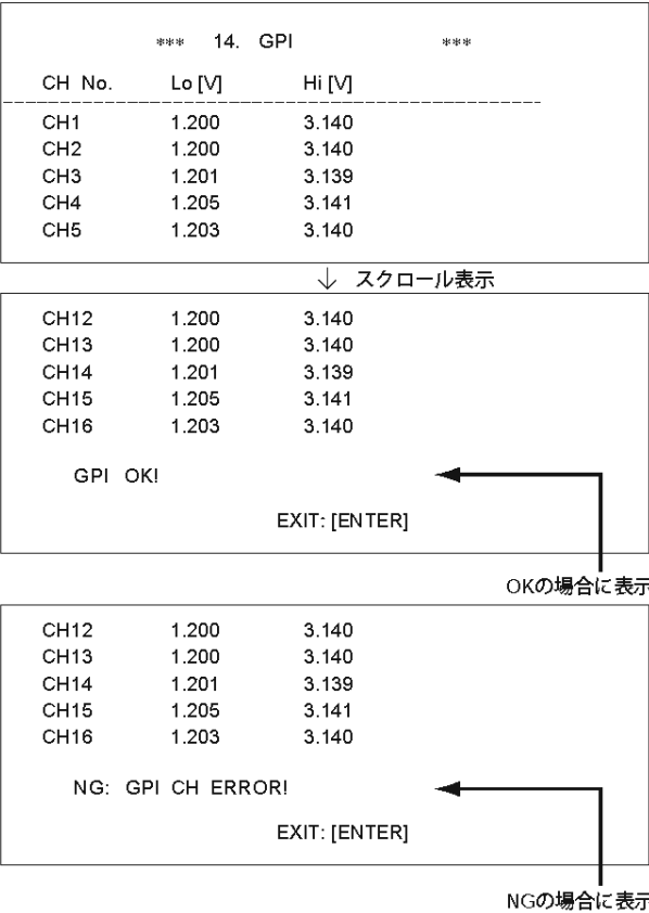
図 34.GPI 検査用画面 (2)
