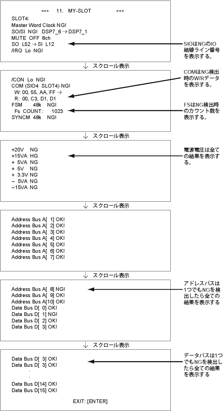
図 26.MY-SLOT 検査用画面 (2)
