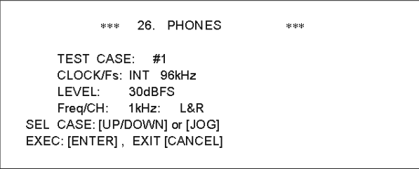
図 49.PHONES 検査用画面 (1)
