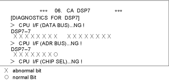
Fig. 19. CA DSP7 Test Screen (2)
