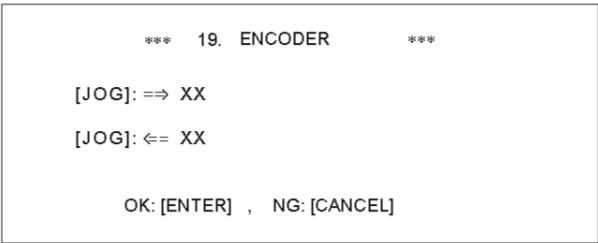
図 40.ENCODER 検査用画面
