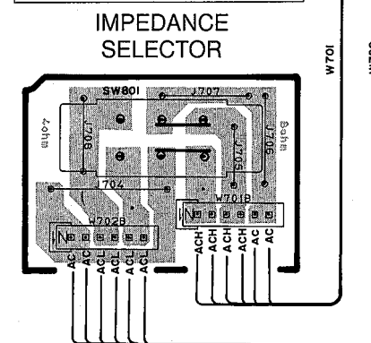
P. C. B. MAIN (4)
