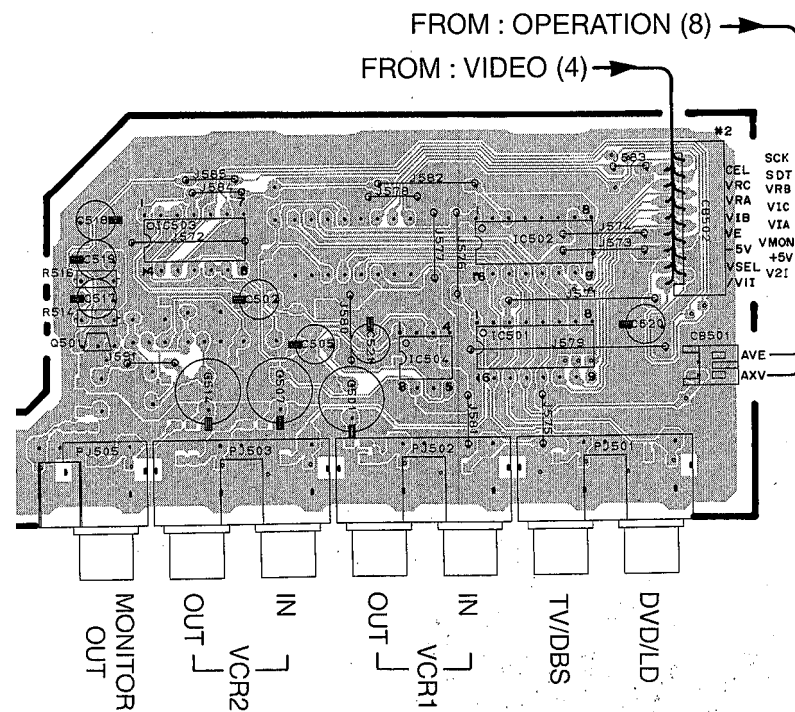
P. C. B. VIDEO (3)
