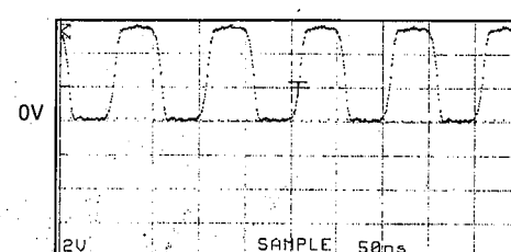
Point ⑦ (Pin16 of IC4)
