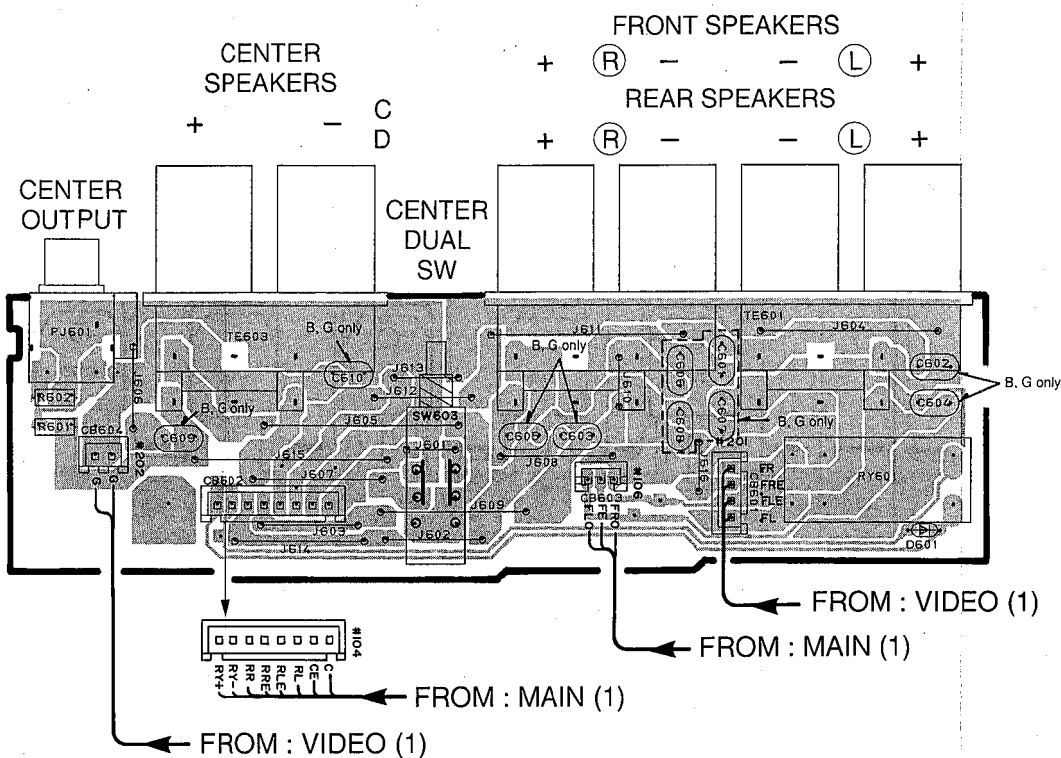
P. C. B. MAIN (2)
