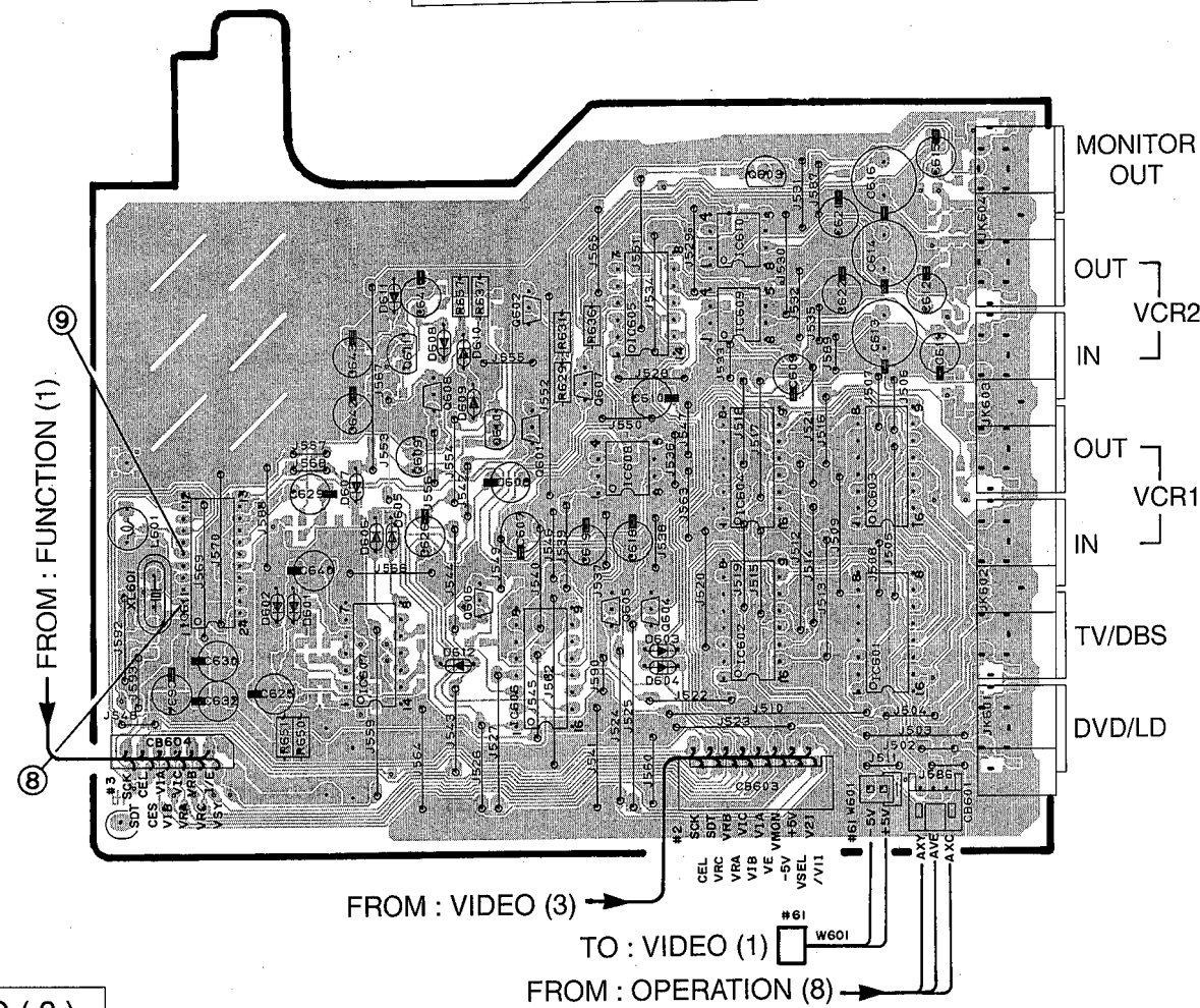
P. C. B. VIDEO (4)
