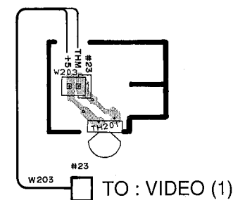
P. C. B. VIDEO (2)
