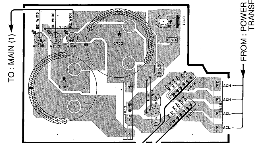
P. C. B. MAIN (3)
