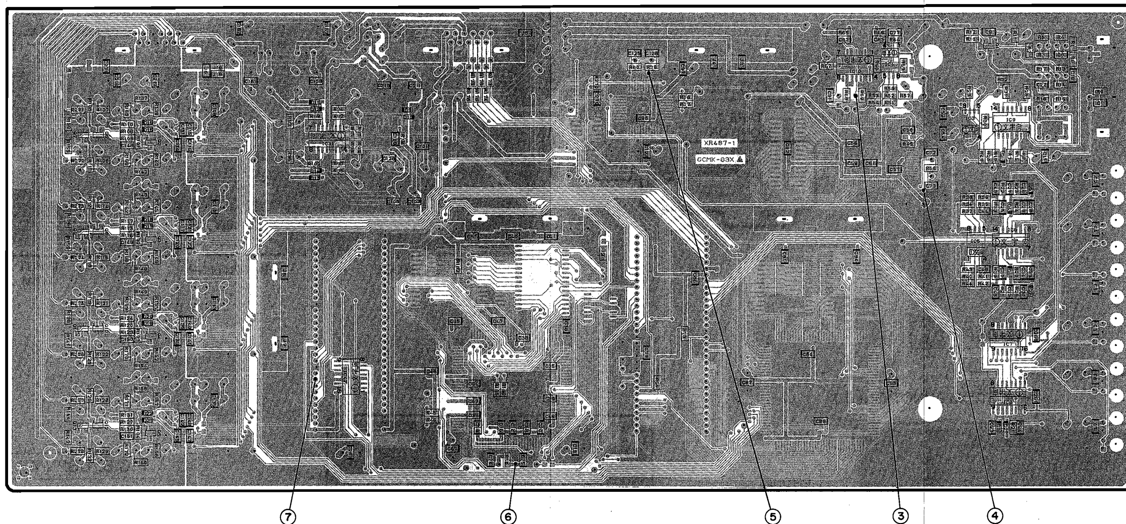
P.C.B. DSP ( 1 )
