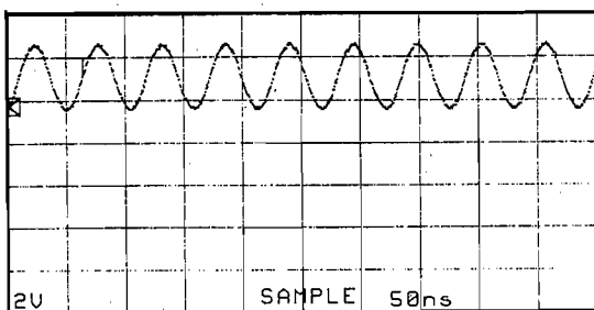
Point ④ (Pin 3 of IC 11)
