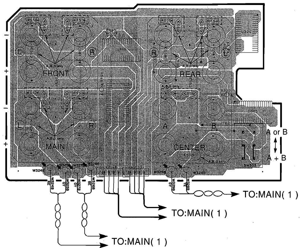
P.C.B. MAIN ( 2 )
