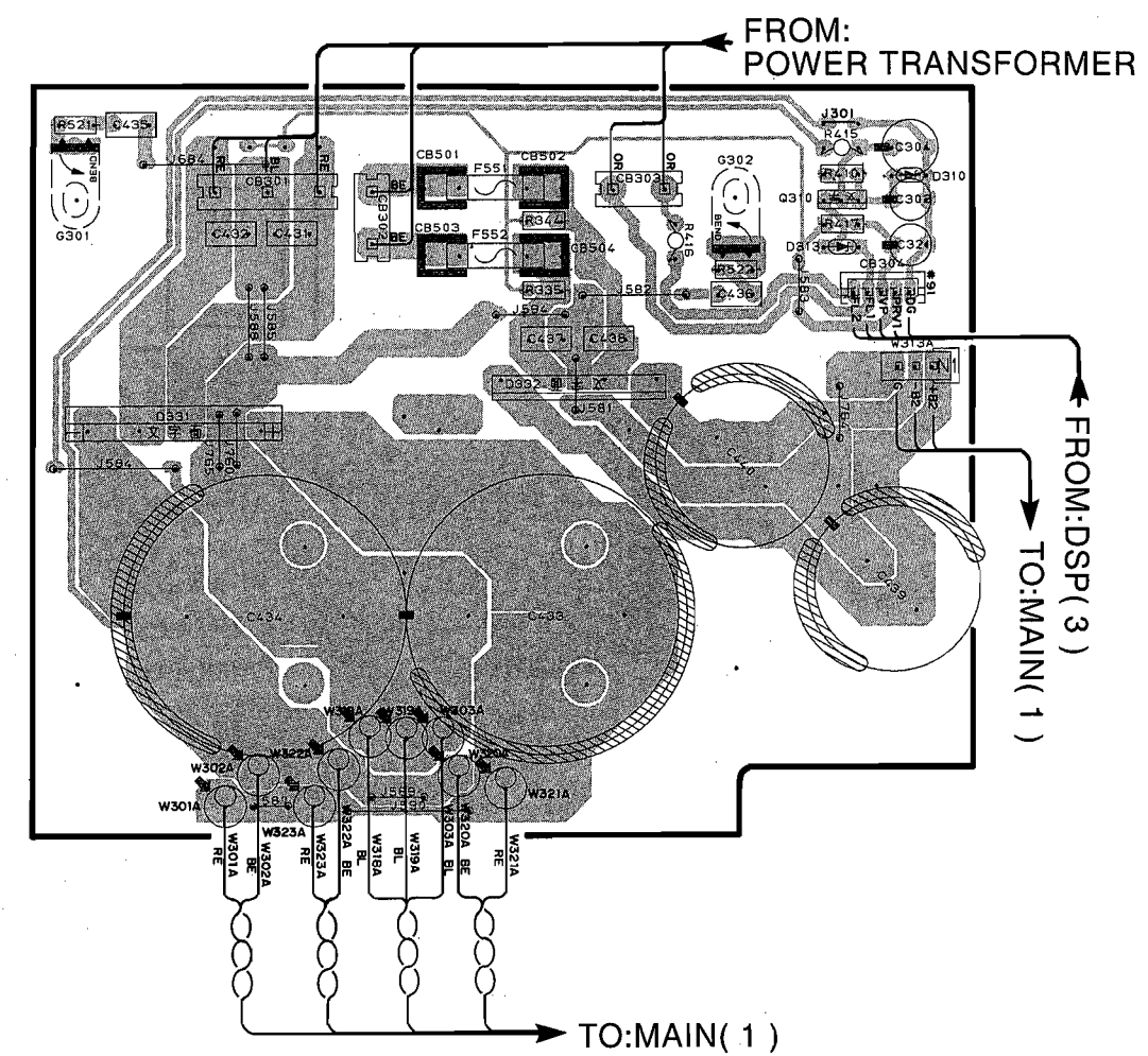
P.C.B. MAIN ( 3 )
