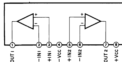
IC904 : NJM2068LD Dual OP-Amp
