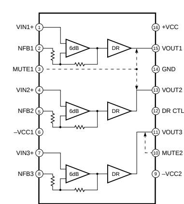
IC711 : LA7104M Double Scart Interface
