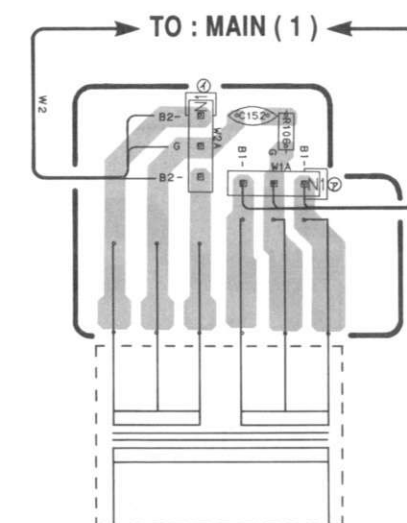
P.C.B. MAIN ( 2 )
