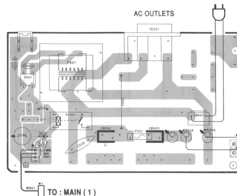
P.C.B. FUNCTION ( 3 )
