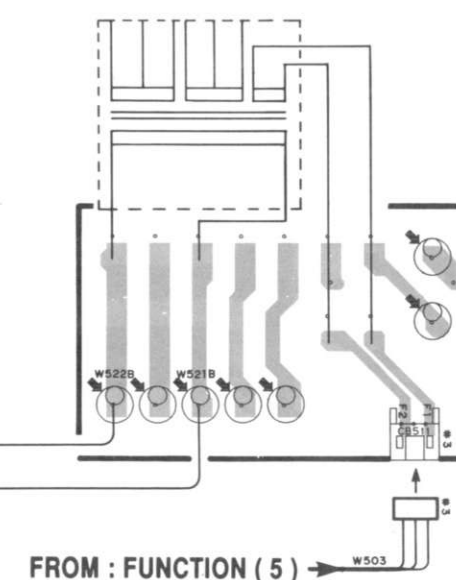
P.C.B. FUNCTION ( 4 )
