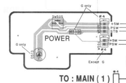
P.C.B. FUNCTION ( 7 )
