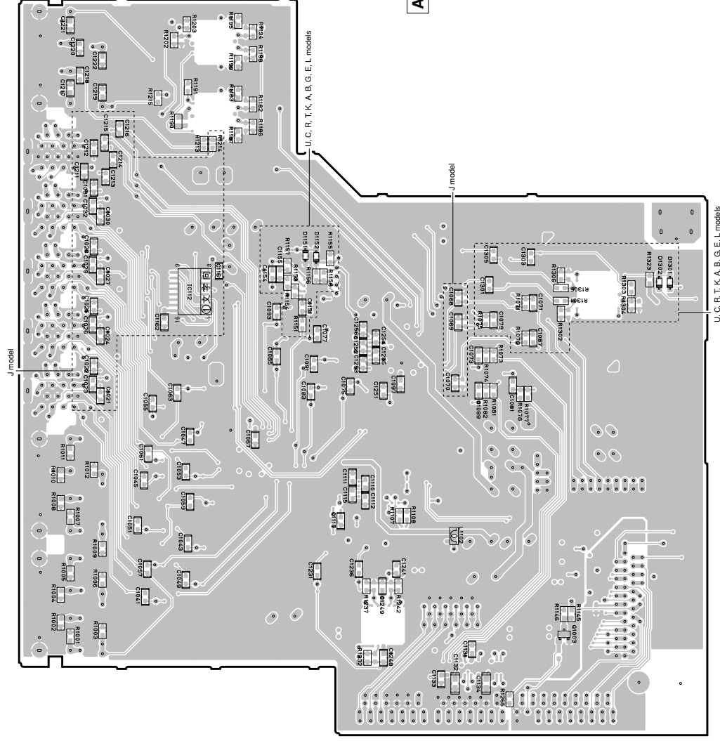
AVIDEO (3) P.C.B.
