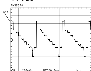
TP 6 : Y_ENC
