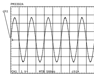
TP 14 : ANALOG OUTPUT AUDIO HP_R &amp; HP_L
