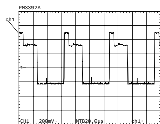
TP 2 : video G
