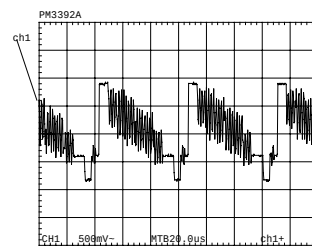
TP 19 : CVBS_OUT
