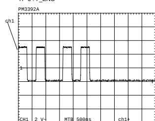
TP 7 : PCM_OUT0
