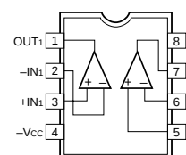
IC1, 2, 7 : KIA4558P Dual OP-Amp
