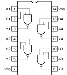
IC312 : TC74HCT00AF Quad 2 Input NAND
