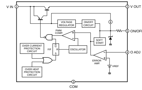
IC275 : PQ1CG21H2F IC276 : PQ1CG2032FZH Voltage Regulator
