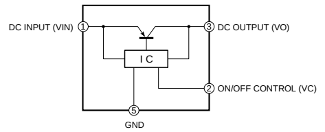
IC1 : PQ012FZ012P Regulator
