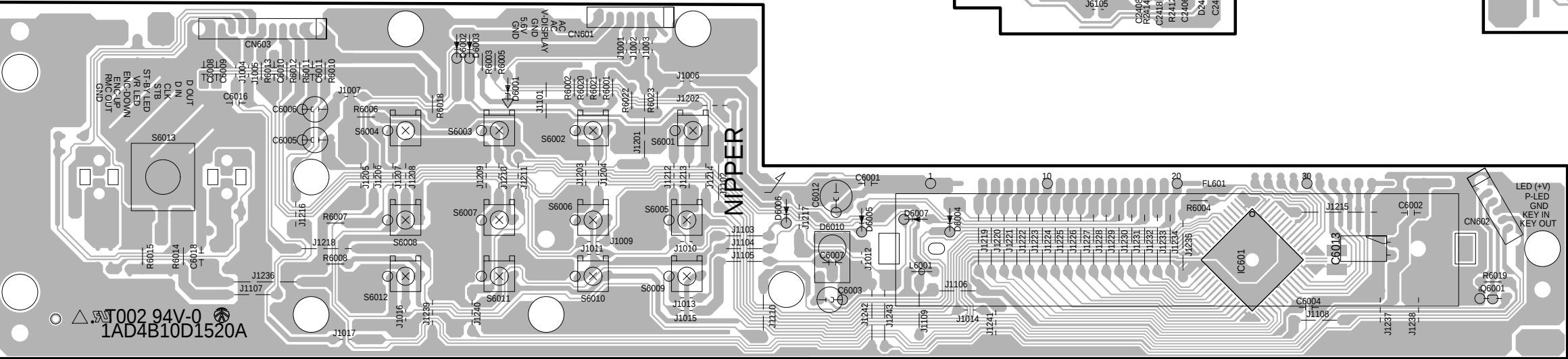
FRONT P.C.B.
