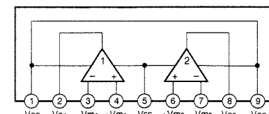
IC217 : BA15218N Dual OP-Amp
