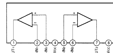
IC217 : BA15218N Dual OP-Amp
