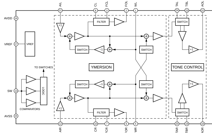
IC814 : YSS247-D YMERSION
