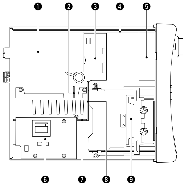
Top side
