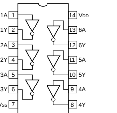
IC10 : TC74HC04AF Hex Inverters
