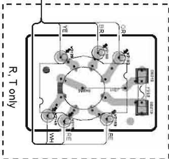
P.C.B. MAIN (4)
