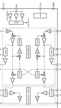
IC811 : VS2820 YMERSON
