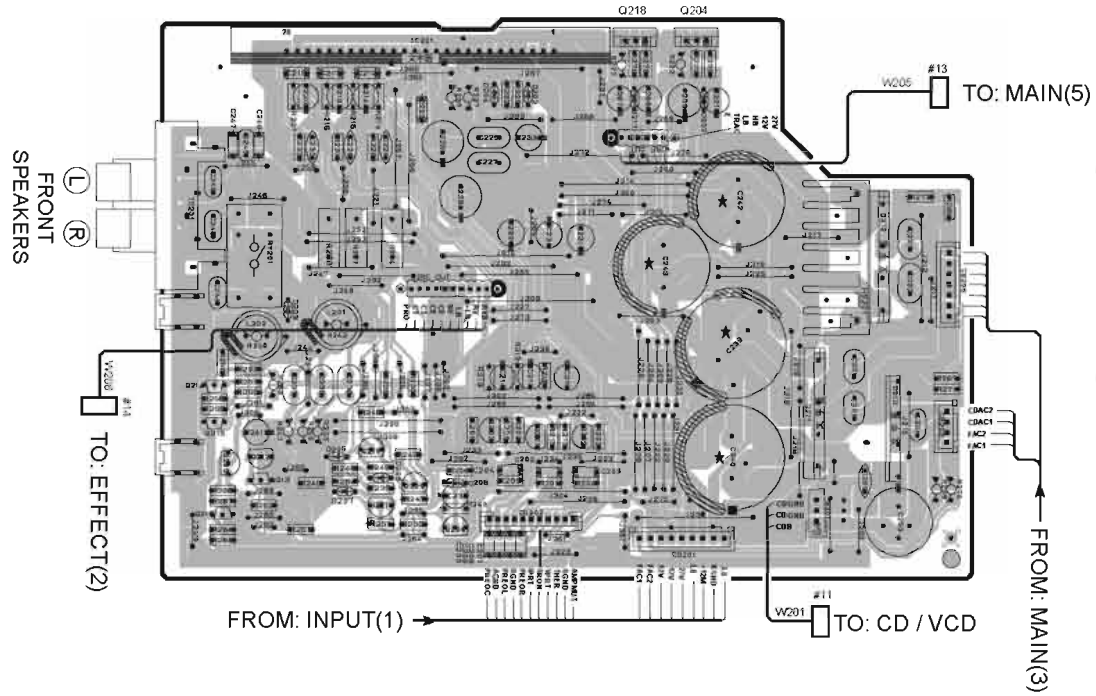
P.C.B. MAIN(1)
