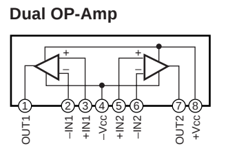
IC104 : NJM2068LD IC107-109 : M5220L Dual OP-Amp
