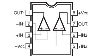
IC813-817: M5220FP
