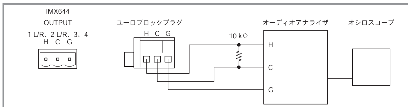
図 5 : OUTPUT 1 L/R、2 L/R、3、4 接続
