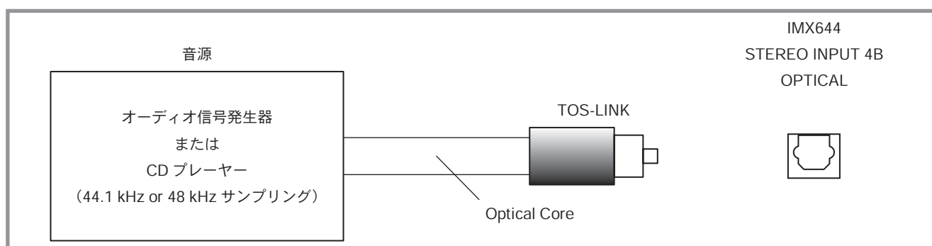
図 4 : STEREO INPUT 4B 接続
