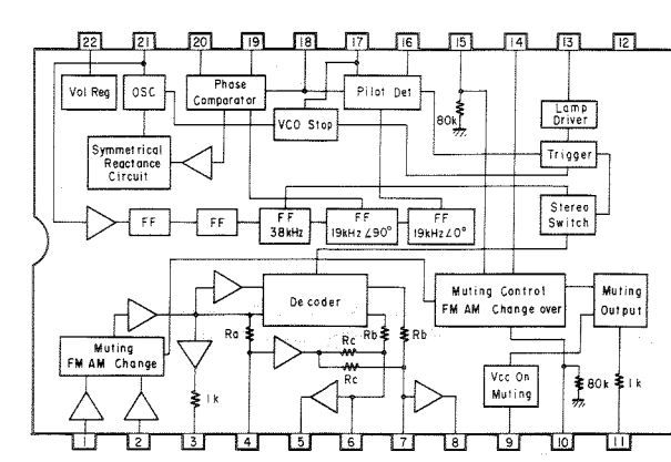
IC3 : LA3401 MPX
