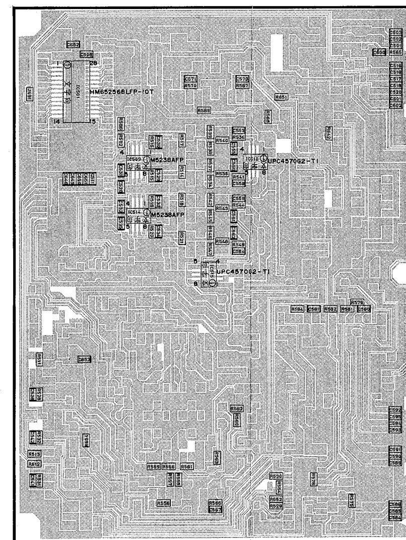
RX-V1070/V870 DSP P. C. B. ( 1 )
