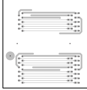
FL (3) P.C.B. (Side B)
