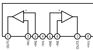
IC701 : NJM2068L-D Dual OP-Amp
