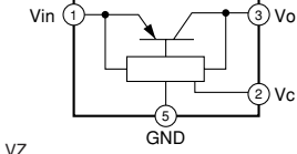
IC803: PQ025EZ5MZP Regulator
