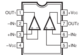
IC813-817: M5220FP
