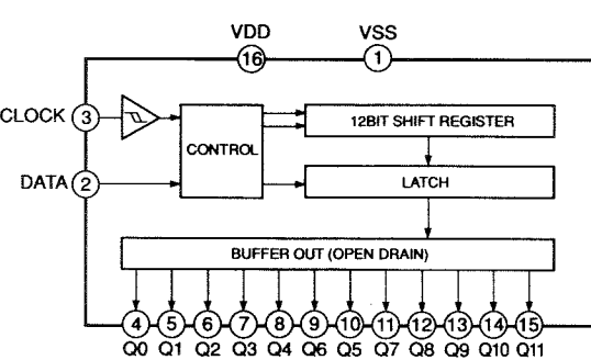
IC504 : BU2040 Port Expander
