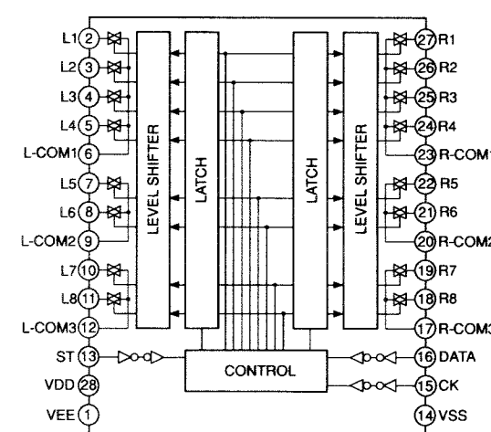
IC502 : NJU7313 Analog Function Switch
