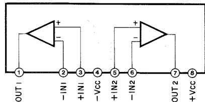
IC501, 503 : NJM2068L-D Dual OP-Amp
