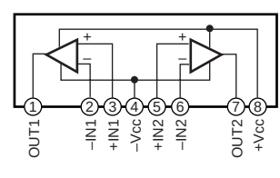
IC104 : NJM2068LD IC107-109 : M5220L Dual OP-Amp
