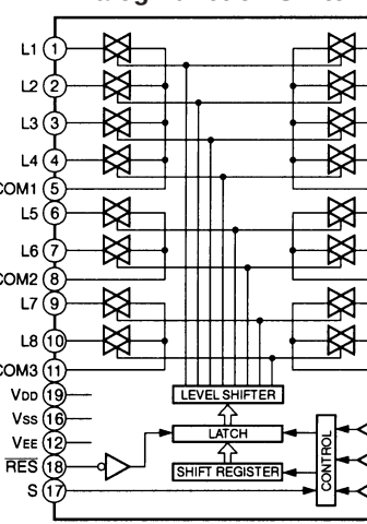
IC101 : LC78211 Analog Function Switch
