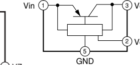
IC803: PQ025EZ5MZP Regulator
