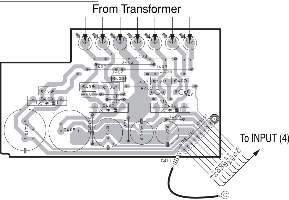
INPUT (5) P. C. B.
