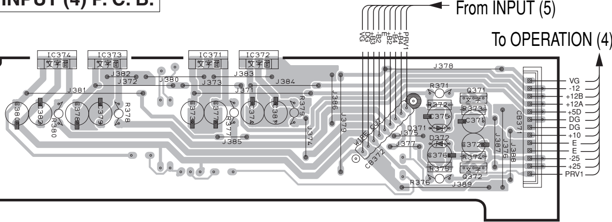
INPUT (4) P. C. B.
