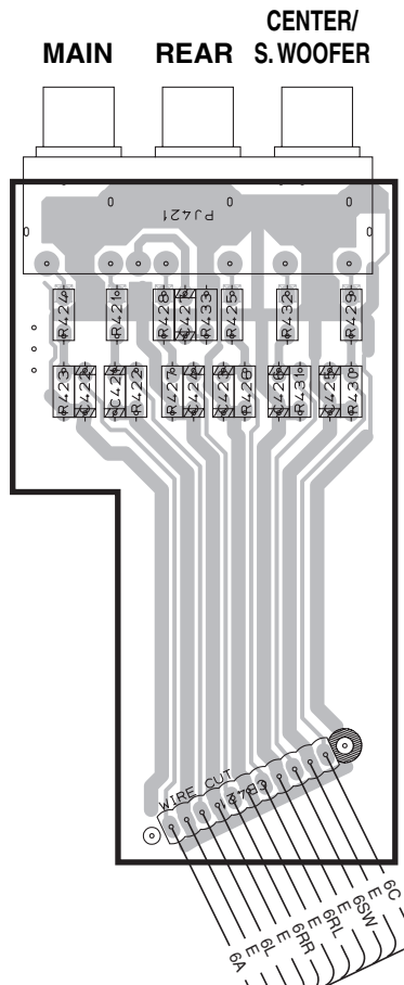
INPUT (6) P. C. B.
