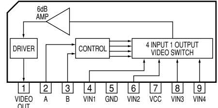
IC551: LA7956
