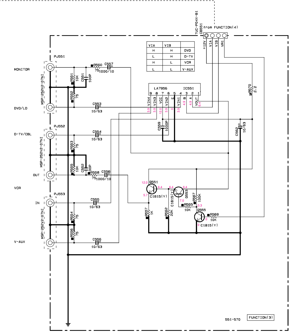
IC551: LA7956
