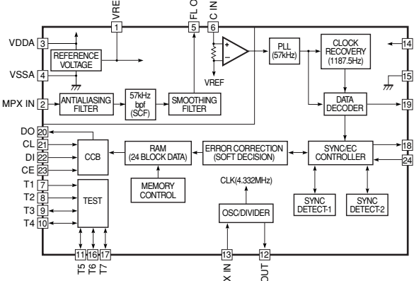
IC571: LC72722
