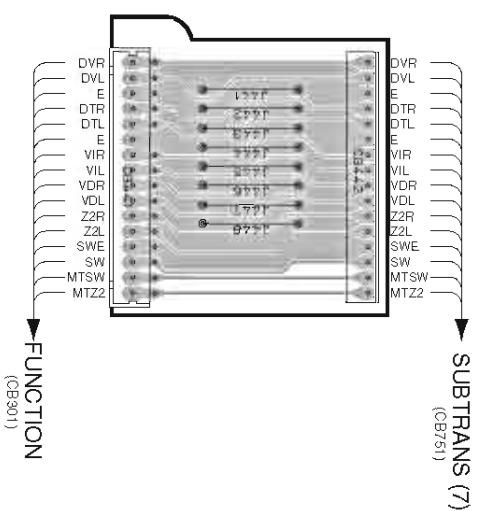
SUBTRANS (9) P.C.B.
