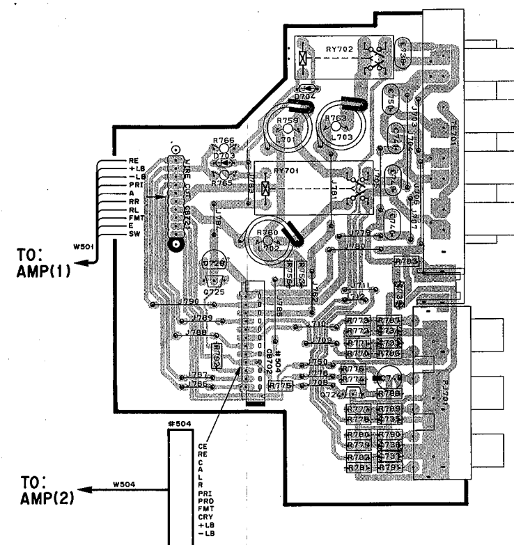
AMP P. C. B. (3)
