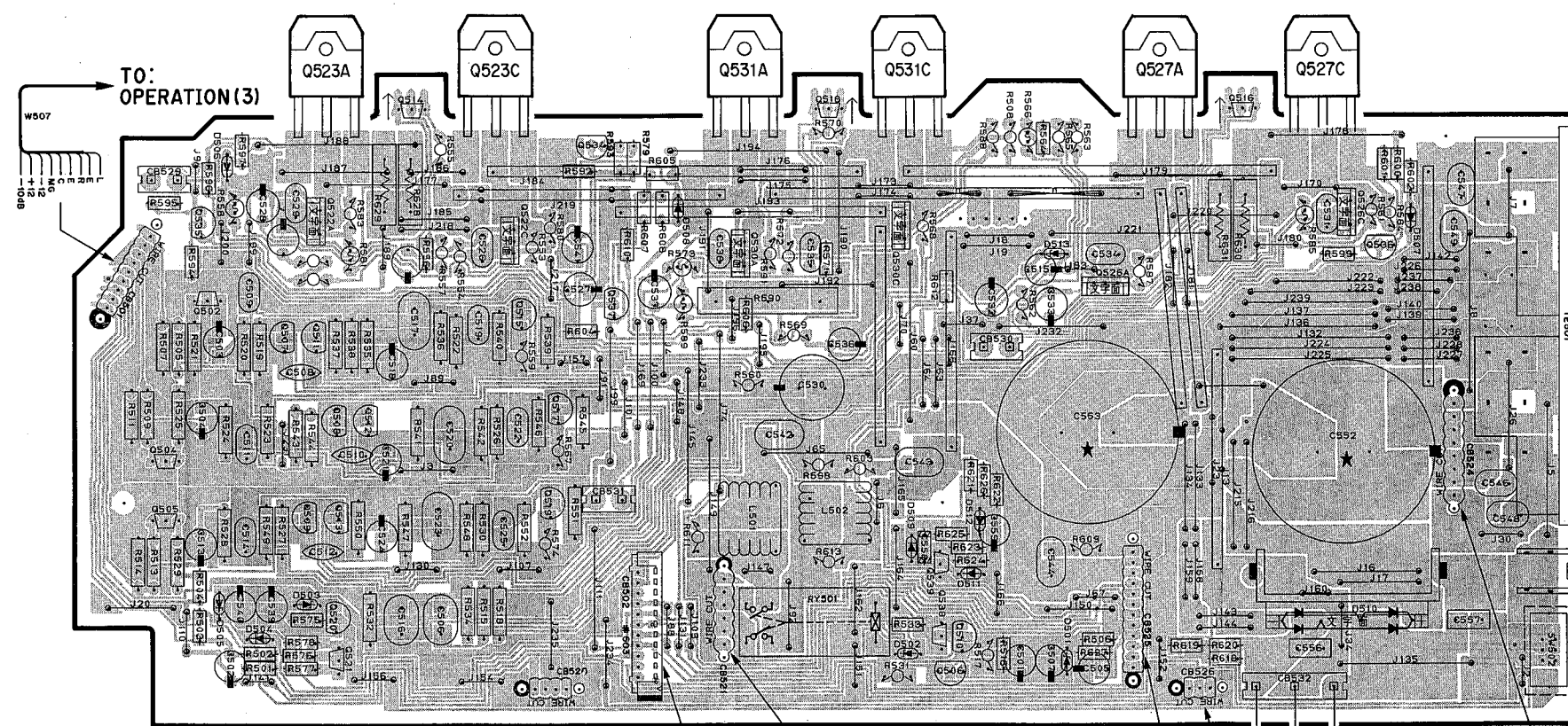
AMP P. C. B. (1)
