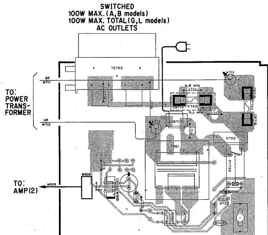
INPUT P. C. B. ( 4 )
