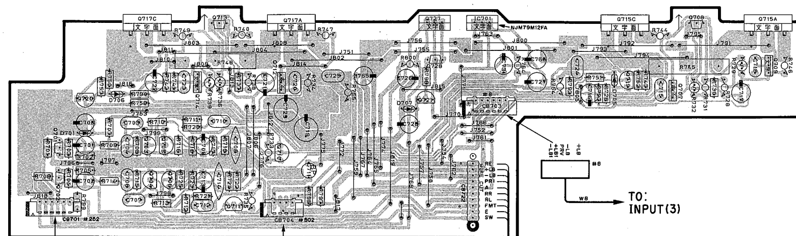
AMP P. C. B. (2)
