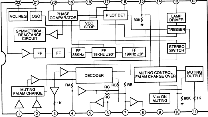
IC4 : LC72720N RDS Decoder
