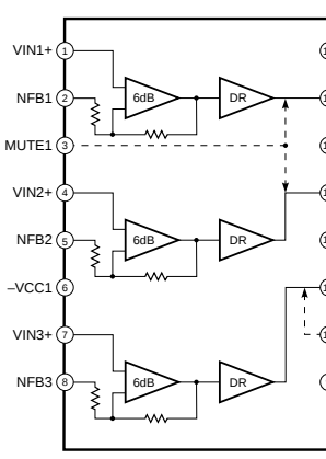
IC711 : LA7104M Double Scart Interface
