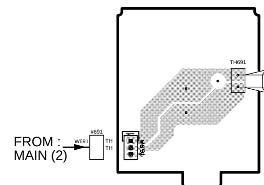
P.C.B. MAIN (7)
