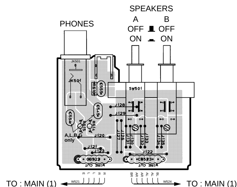
P.C.B. MAIN (4)
