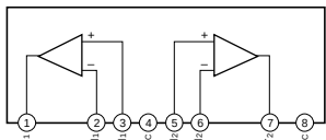
IC201 : NJM2068LD Dual OP Amp
