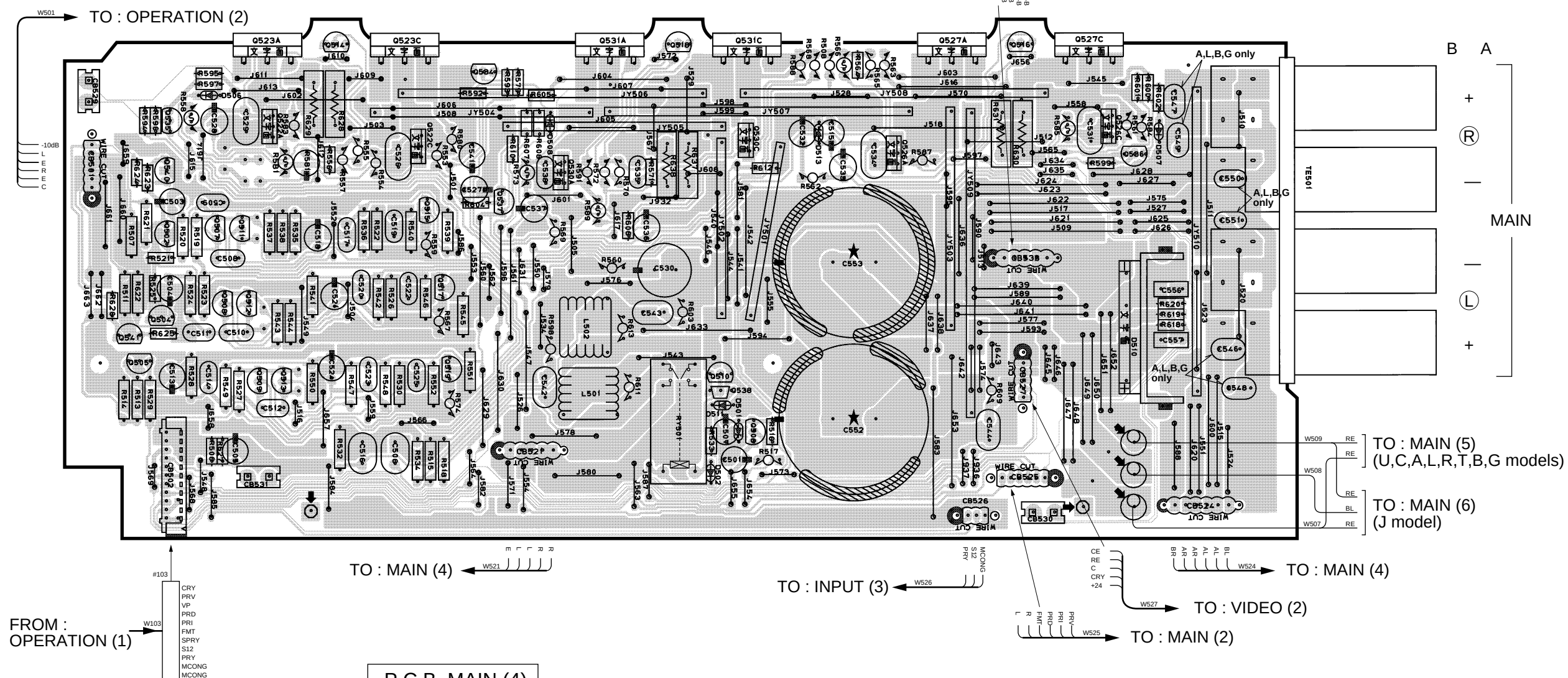
P.C.B. MAIN (4)
