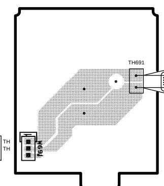
P.C.B. MAIN (7)
