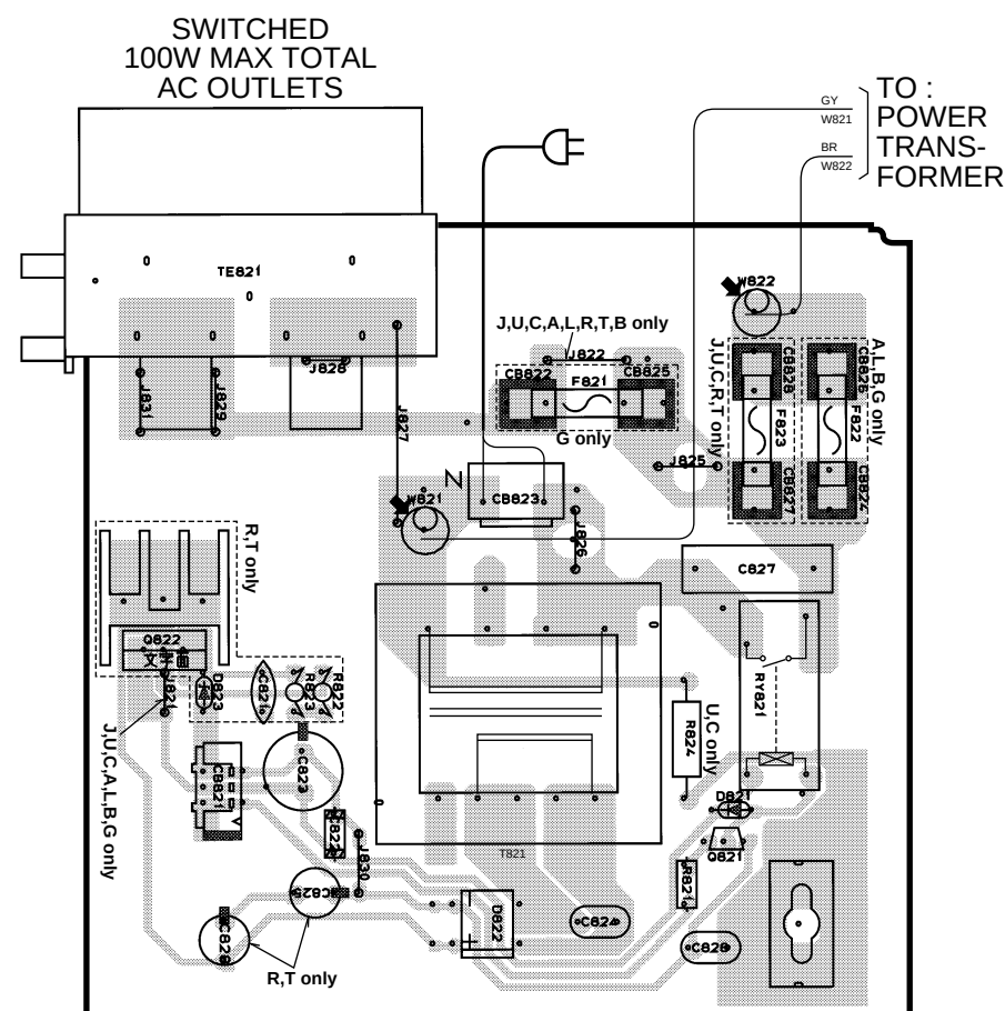
P.C.B. INPUT (3)
