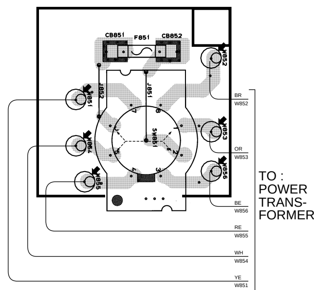
P.C.B. INPUT (4)
