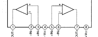
IC201 : NJM2068LD Dual OP Amp
